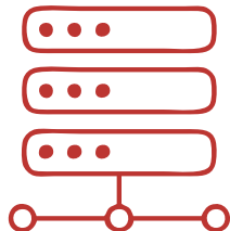
Подсистема «ОБУЧАЮЩИЕСЯ»
