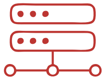
Подсистема «ПРИЁМ»
